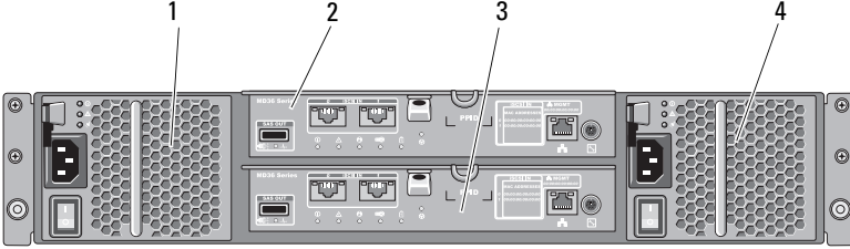
Şekil 2-4. Arka Panel Özellikleri ve Göstergeleri—Dell PowerVault MD3600i Serisi Depolama Dizisi
