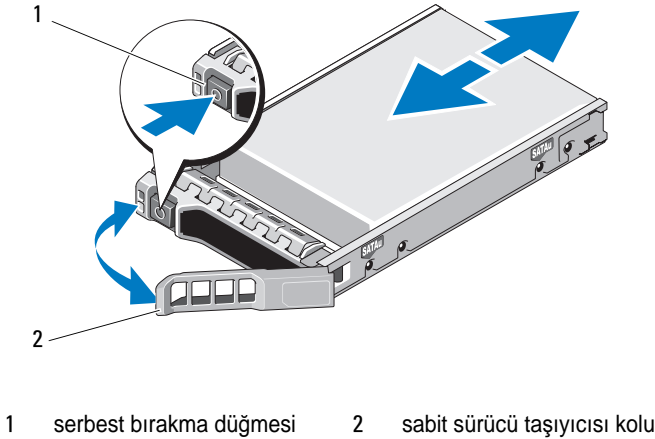
Şekil 16-4. Sabit Sürücüyü Çıkarma ve Takma
