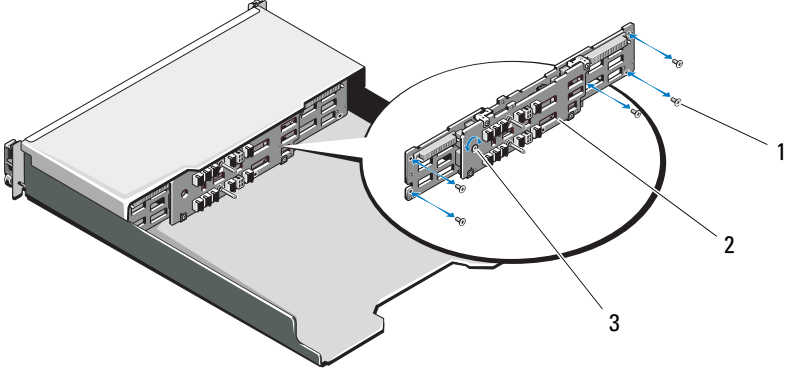
Şekil 16-16. Arka Paneli Çıkartma ve Takma-PowerVault MD3600i
