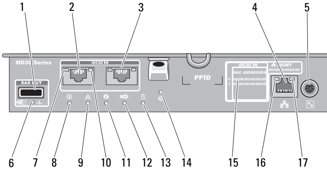
Şekil 3-1. MD3600i Serisi iSCSI RAID Denetleyici Modülü
