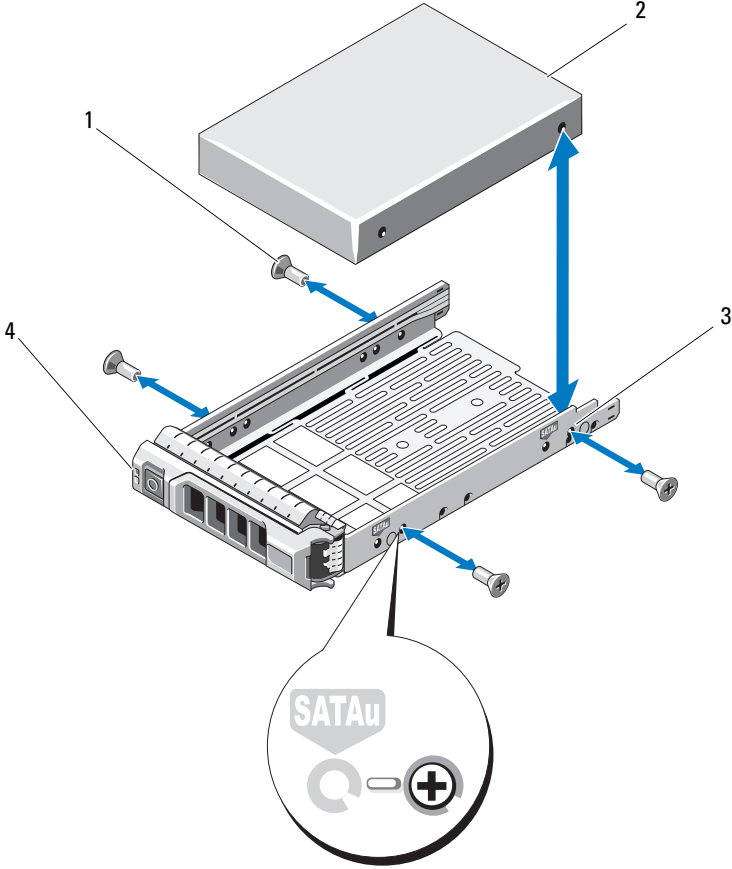
Şekil 16-5. 3,5 İnc Sürücü Taşıyıcıdan Sabit Sürücü Çıkartma ve Takma
