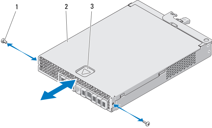
Şekil 16-9. RAID Denetleyici Modülünü Açma ve Kapatma
