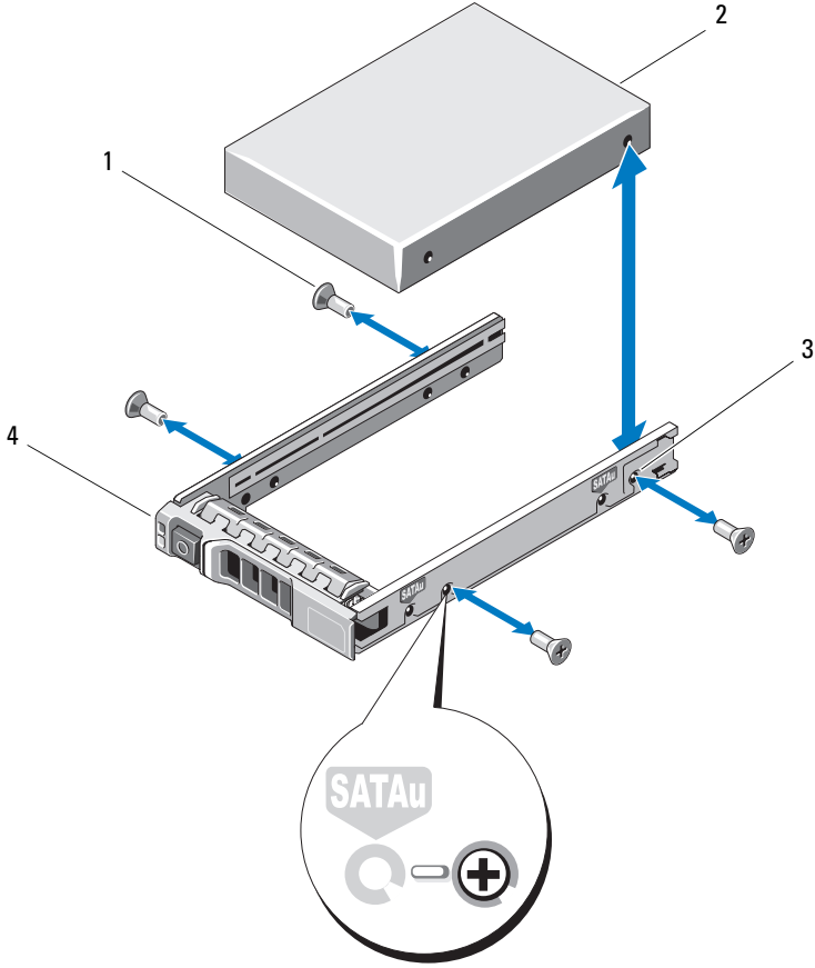
Şekil 16-6. 2,5 İnç Sürücü Taşıyıcıdan Sabit Sürücü Çıkartma ve Takma
