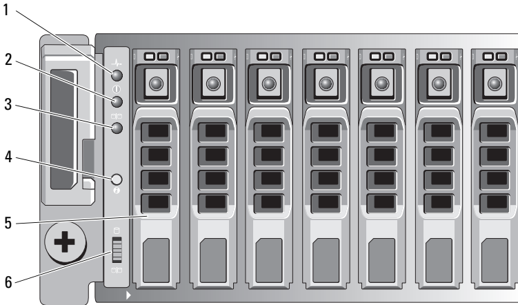
Şekil 2-2. Ön Panel Özellikleri ve Göstergeleri—Dell PowerVault MD3620i
