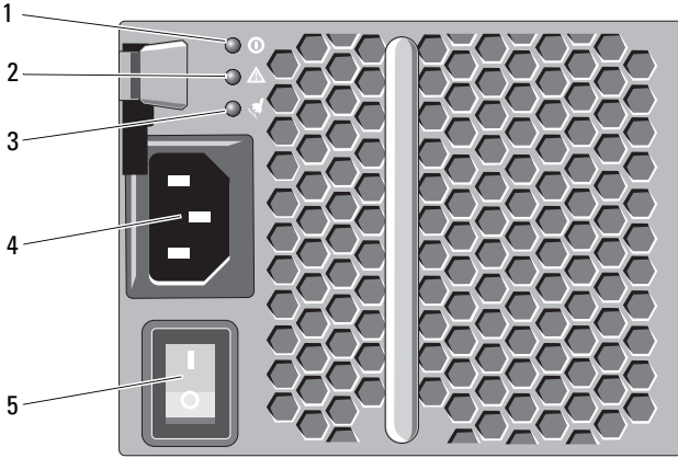
Şekil 2-6. Güç Gösterge Kodları ve Özellikleri
