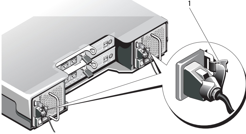
Şekil 16-12. Güç Kablosunun Sabitlenmesi
