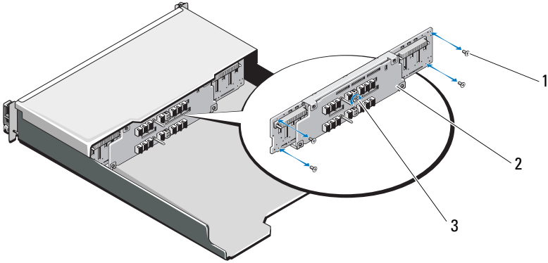
Şekil 16-17. Arka Paneli Çıkartma ve Takma-PowerVault MD3620i
