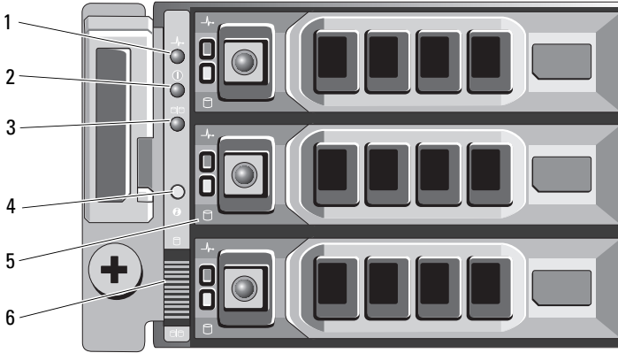
Şekil 2-1. Ön Panel Özellikleri ve Göstergeleri—Dell PowerVault MD3600i
